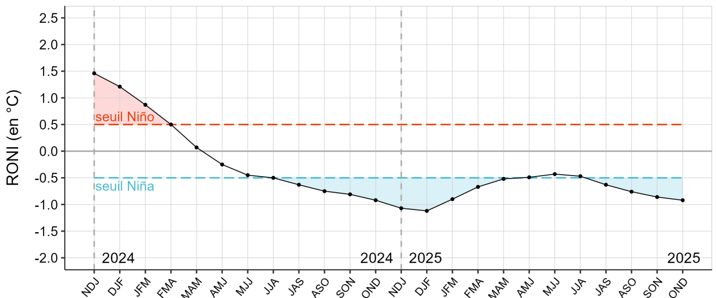
Indice océanique relatif Niño 3.4 (RONI) au cours des 24 derniers mois
